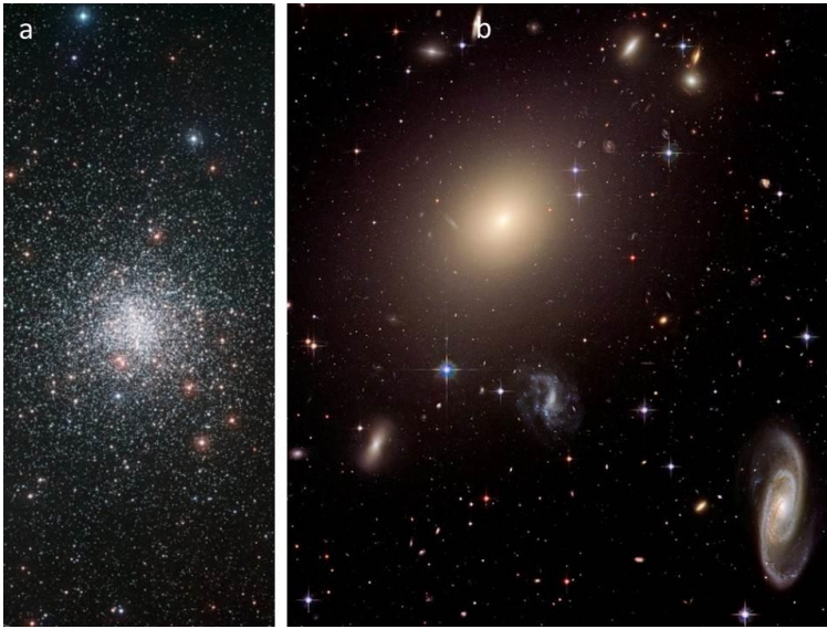
Илл. 1 (а). Шаровое скопление звезд М4 с радиусом в 35 световых лет, расположенное на расстоянии в 7200 св. лет (фото ESO); (б). Кластер галактик Abel S740 (NASA, ESA, STScI/AURA, J. Blakeslee). Эллиптическая галактика ESO 325-G004 (выше и левее центра) имеет размер больше 100 тысяч св. лет и расположена на расстоянии около 420 миллионов св. лет; в правом нижнем углу - спиральная галактика.
