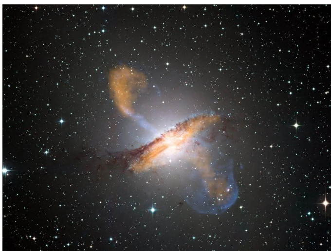
Илл. 8 Галактика Центавр А на расстоянии 10-16 млн. св.лет. В центре диска расположена черная дыра в 55 миллионов солнечных масс, выбрасывающая в противоположных направлениях два огромных джета (ESO/WFI (Optical); MPIfR/ESO/APEX/A.Weiss et al. (Submillimetre); NASA/CXC/CfA/R.Kraft et al. (X-ray)).
